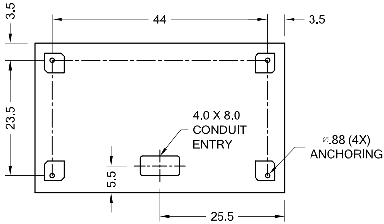
VIEW A-A
